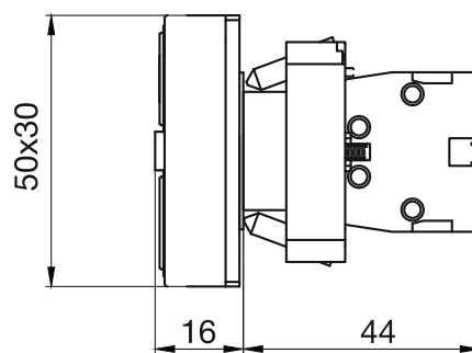
Двойная «ПУСК-СТОП»
